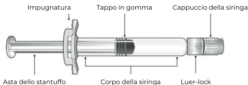
Figura 1: componenti della siringa Luer-lock
